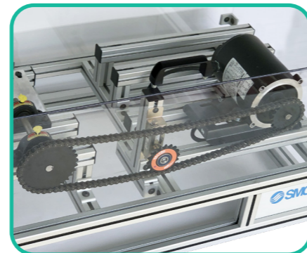
*Sistema de entrenamiento de transmisión de cadena
